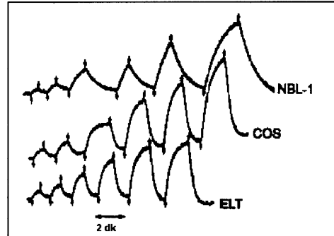
Şekil 6. Değişik LA konsantrasyonlarında (1, 2, 5, 10, 20, 30 mmol) COS, NBL1 ve ELT hücrelerine LA taşınımı esnasında sitozolik pH değişim grafikleri (grafik pH değişimine duyarlı floresan maddenin 440/490 nm'deki absorpsiyon değişimlerini göstermektedir) (Wilson ve ark., 1998).
