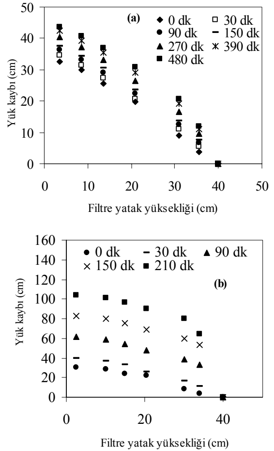
Şekil 5. Filtre yatağı boyunca yük kaybı gelişim eğrileri (a) 5.60 m/saat filtre hızı ve 0.5 mg Fe(II)/L, (b) 5.60 m/saat filtre hızı ve 5.0 mg Fe(II)/L
