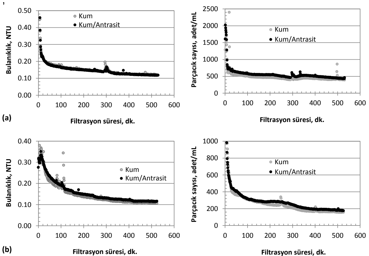
Şekil 4. Filtre çıkış suyu bulanıklık ve parçacık sayısı değişimi (İkitelli Arıtma Tesisi giriş suyu, a) 10 mg/L alum b) 5 mg/L demir klorür)
