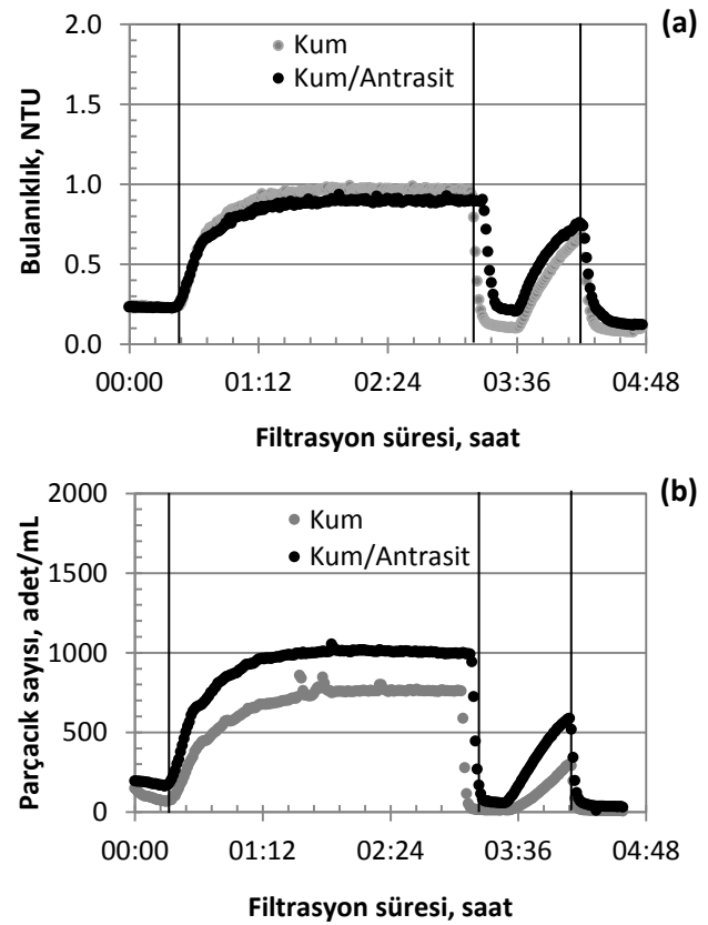
Şekil 2. Sentetik su ile yürütölen filtrasyon deneyi çıkış suyu kalitesi değı şimi
