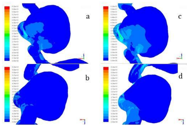
Şekil 7. Anevrizma boyunca duvar kayma gerilmeleri. a ve b newtoniye, c ve d ise Carreau akışkanları göstermektedir. a ve c tepeden, b ve d ise aşağıdan görünüştür.
