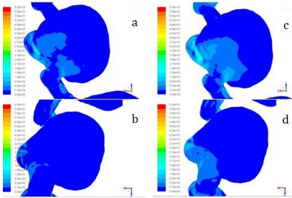
Şekil 6. Anevrizma boyunca duvar kayma gerilmeleri. a ve b newtoniye, c ve d ise power law akışkanları göstermektedir. a ve c tepeden, b ve d ise aşağıdan görünüştür.
