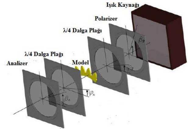
Şekil 1. Dairesel polariskop [17]
