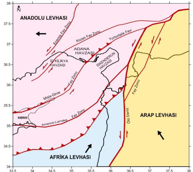
Şekil 2. Çalışma alanı ve çevresinin güncel tektonik haritası [3, 7].
