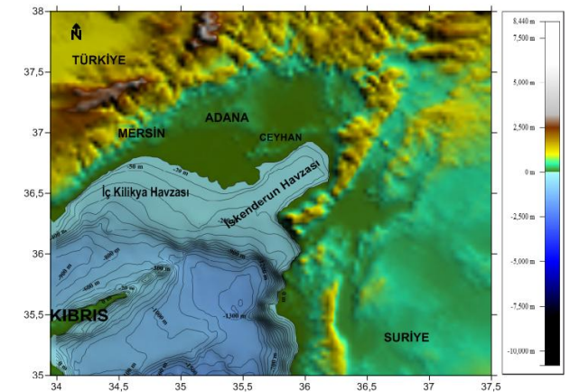
Şekil 3. Çalışma alanının batimetrisi
