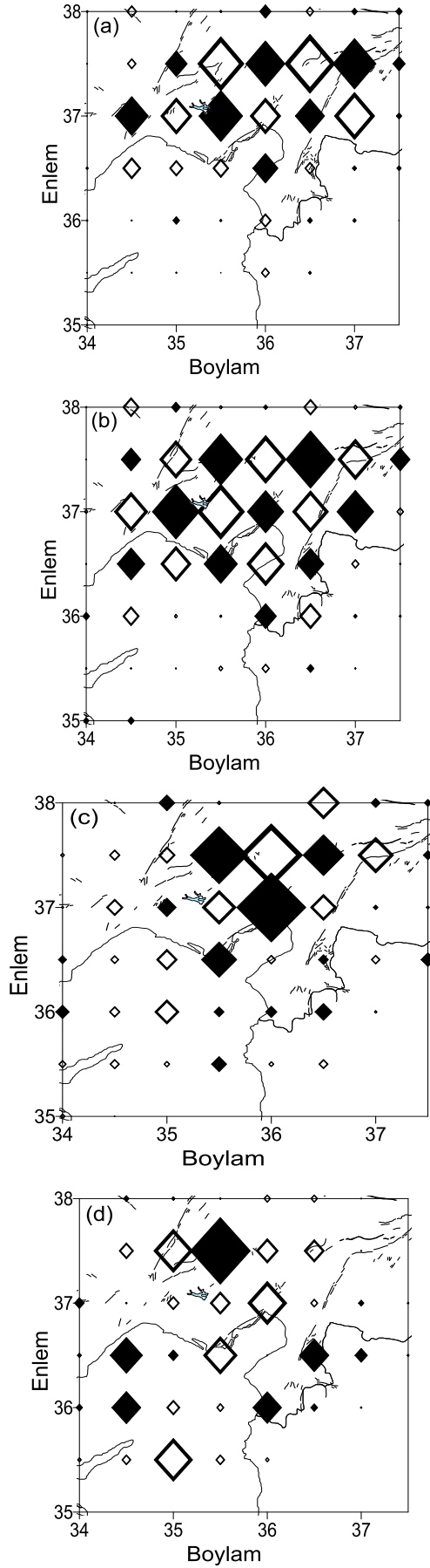
Şekil 8. Dört farklı derinlik için P- dalgası hızı için ters çözüm testi sonucu. Siyah ve beyaz semboller sırasıyla yüksek ve düşük hızları göstermektedir. Değişim ölçeği altta gösterilmiştir (a) 4 km, (b) 8 km, (c) 15 km (d) 25 km
