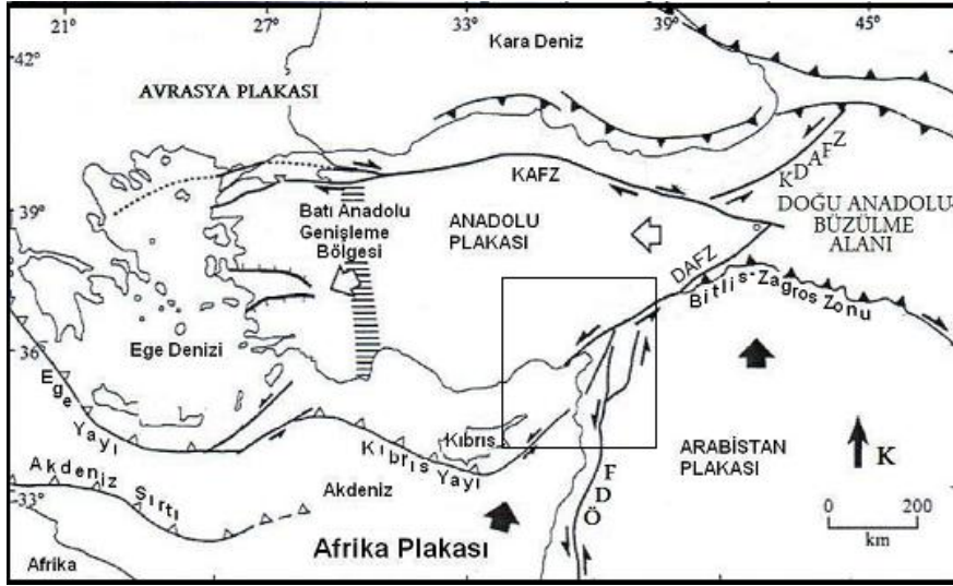
Şekil 1. Türkiye'nin basitleştirilmiş tektonik haritası [3, 8]. ÖDFZ – Ölü Deniz fay zone, DAFZ – Doğu Anadolu Fay Zonu, KAFZ – Kuzey Anadolu Fay Zonu, KDAFZ – Kuzeydoğu Anadolu Fay Zonu, yarım yön işaretli kalın çizgiler doğrultu atımlı fayları, içi dolu üçgen işaretli kalın çizgiler ters fay ve bindirme zonlarını, boş üçgen işaretli kalın çizgiler bindirme zonlarını göstermektedir. Kalın içi dolu yön işaretleri Afrika ve Arap levhasının, içi boşlar ise Anadolu levhasının hareket yönlerini ifade etmektedir.
