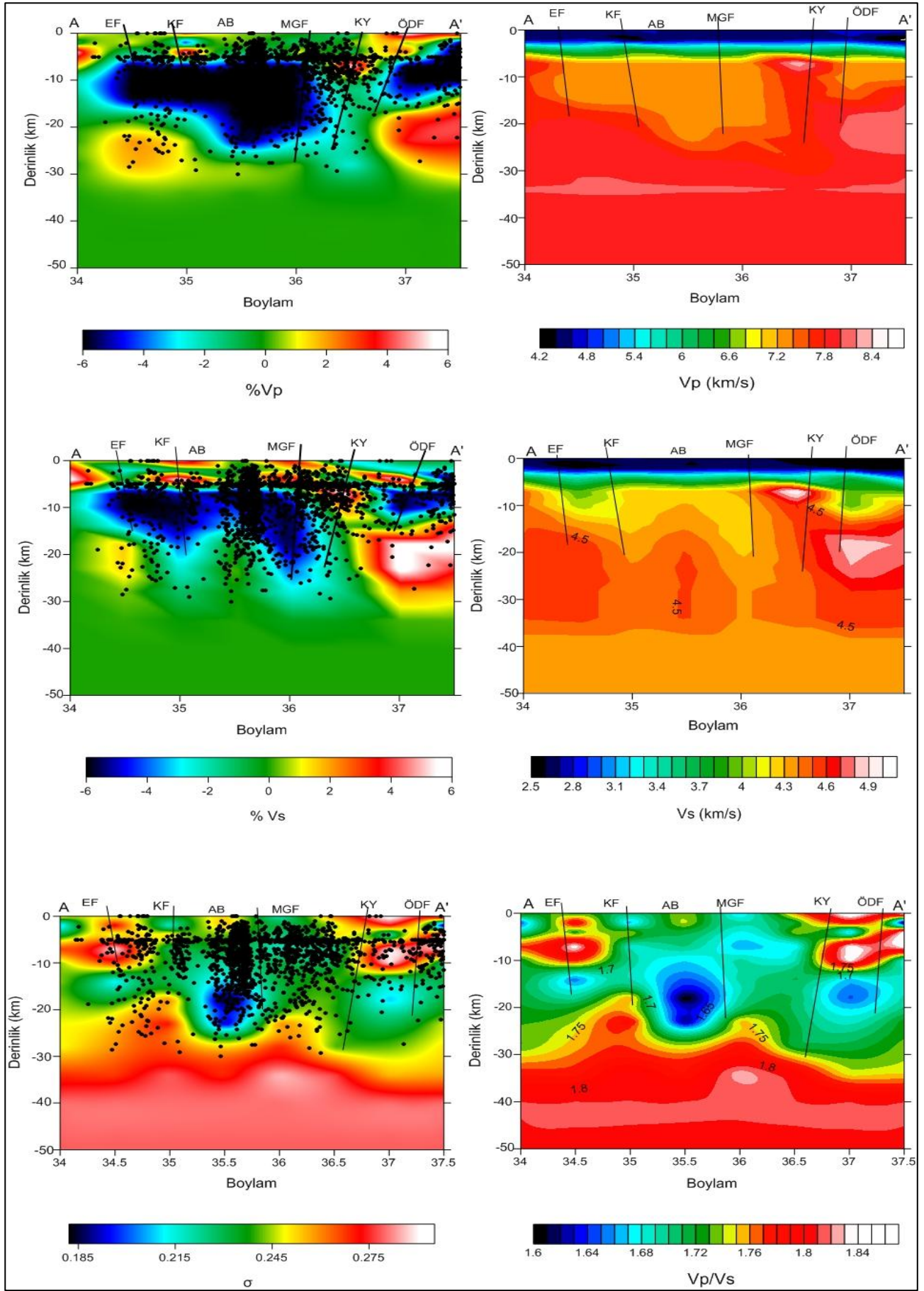
Şekil 12. A-A' doğrultulu hat boyunca Vp, Vs ve \sigma değişimlerine ait derinlik kesitleri EF: Ecemiş Fayı, KF: Kozan Fayı, MGF: Misis-Girne Fayı, KY: Kıbrıs Yayı ve ÖDF: Ölüdeniz Fayı, ALF: Amanos -Larnaka Fayı olarak gösterilmiştir.
