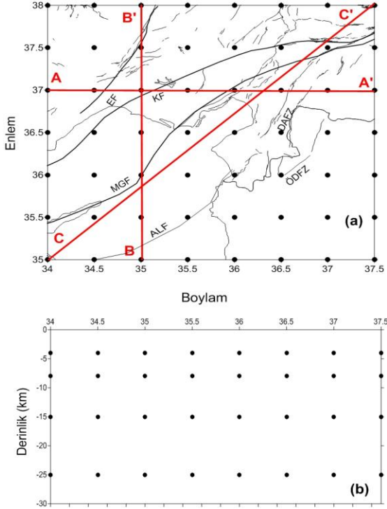
Şekil 6. Yatay yöndeki grid aralıkları konumu ve çalışma alanı içinde alınan kesitler (a) ve düşey yönlerde grid aralıklarının konumu (b) EF: Ecemiş Fayı, KF: Kozan Fayı, MGF: Misis-Girne Fayı, DAFZ: Doğu Anadolu Fay Zonu ve ÖDFZ: Ölüdeniz Fayı, ALF: Amanos -Larnaka Fayı olarak gösterilmiştir.
