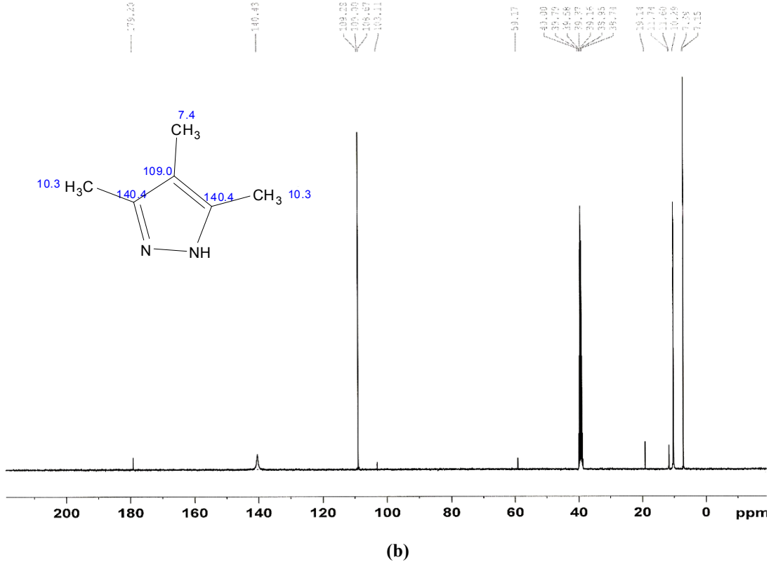
Şekil 5. Tmp'nin DMSO içinde 400 mHz ve 300 K'de a) ^1\text{H} -NMR b) ^{13}\text{C} -NMR spektrumu
