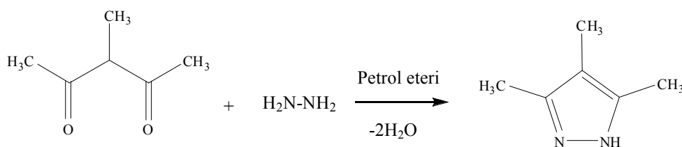
Şekil 4. 3-metil-2,4-pentandion ve hidrazinden tmp sentezi
