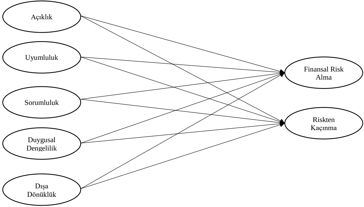
Şekil 1. Araştırma Modeli
