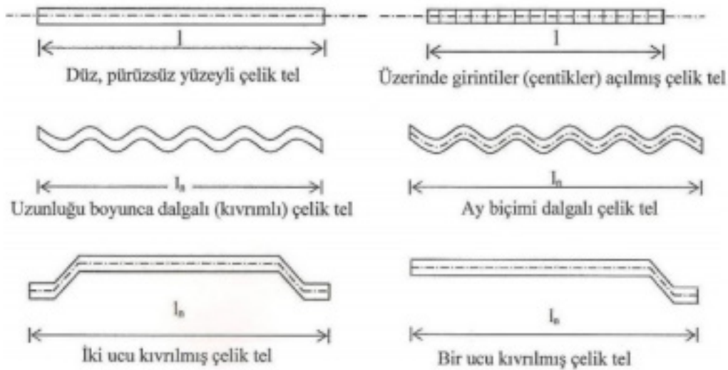
Şekil 1. Çelik liflerin şekilleri (TS 10513, 1992)
