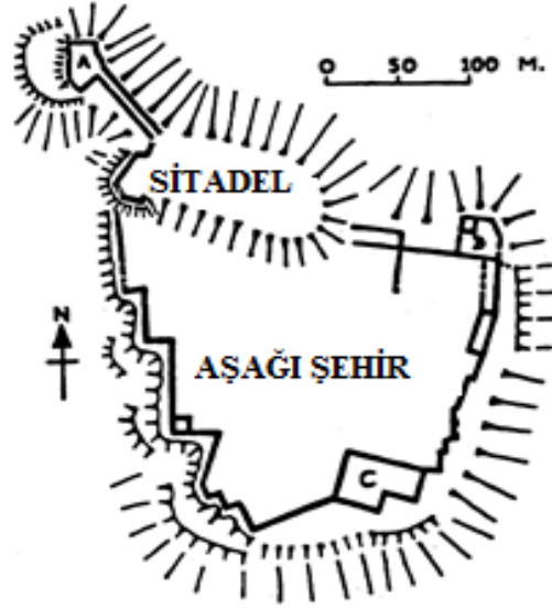
Resim – 1: Kefkalesi Yerleşiminin Planı (Burney, 1957, s. 51 fig. 12’den uyarlama)
