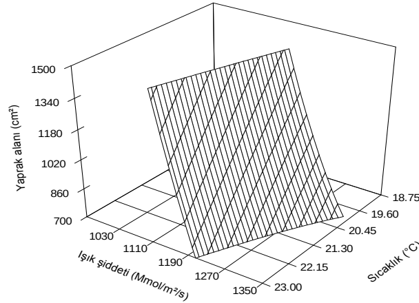
Şekil 1. Işık (Mmol/m 2 /s) ve hava sıcaklığı (°C) bağlı olarak mısırdaki yaprak alanının değişimi Figure 1. Change in leaf area of corn depending on light (Mmol/m 2 /s) and temperature (°C).
