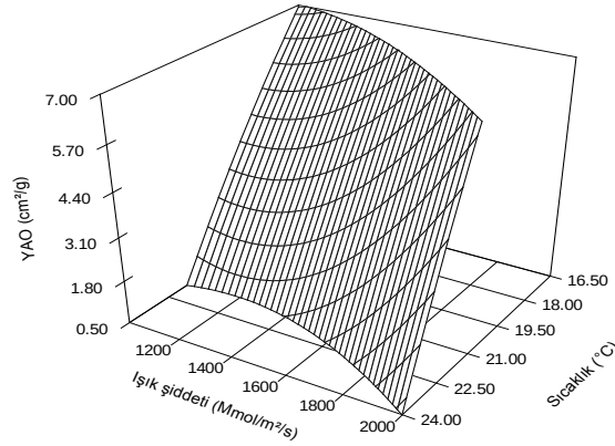
Şekil 4. Işık (Mmol/m²/s) ve hava sıcaklığına (°C) bağlı olarak mısırdaki oransal yaprak alanının değişimi.
