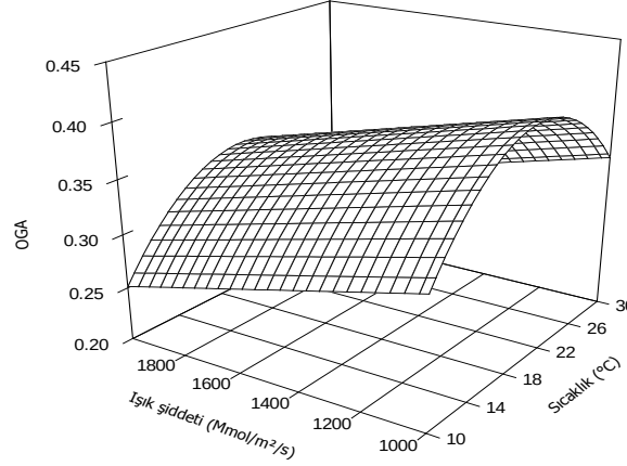
Şekil 8. Işık (Mmol/m²/s) ve hava sıcaklığına (°C) bağlı olarak mısırdaki oransal gövde ağırlığının değişimi.
