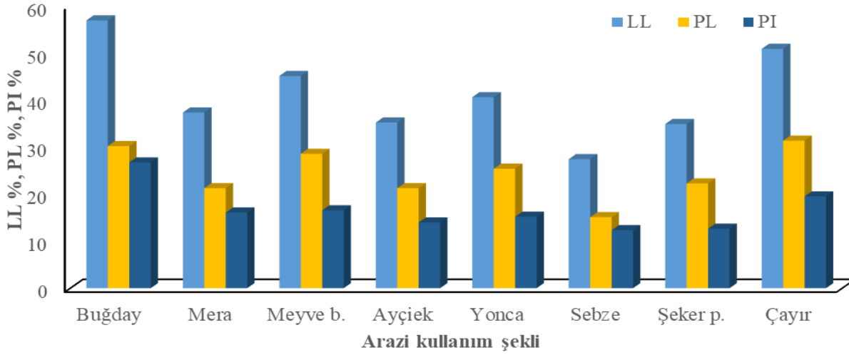
Şekil 1. Arazi kullanım şekli ile kıvam limitleri arasındaki ilişkiler.
