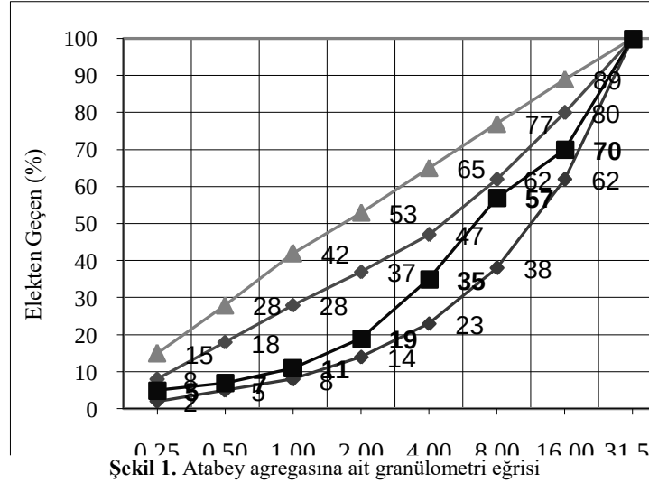
Şekil 1. Atabey agregasına ait granülometri eğrisi
