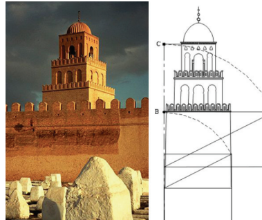
Şekil 8. Kayravan'daki Büyük Cami'nin minaresi için yapılmış altın oran uyum çalışması (Boussora, 2004)
