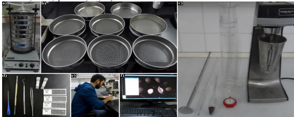
Şekil 5. Sedimantolojik ve paleontolojik analizlerde kullanılan araçlar. a ve b: Restch marka elek seti; c) Hidrometre analizlerinde kullanılan temel araçlar; d) fosillerin ayrılmasında ve depolanmasında kullanılan araçlar; e) Fosillerin ayrılmasında yararlanılan mikroskop; f) Fosillerin fotoğraflanmasında kullanılan kameram yazılımının ekran görüntüsü.
