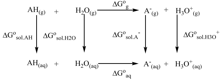
Şekil 2. Asitlik sabit termodinamik çevrimin su fazındaki mekanizması.
