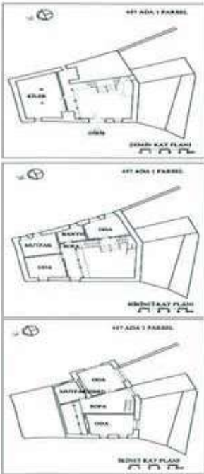
Şek. 8. Taşıklı/dış sofalı bir evin (env. no: J18.B5.869) kat planları.
