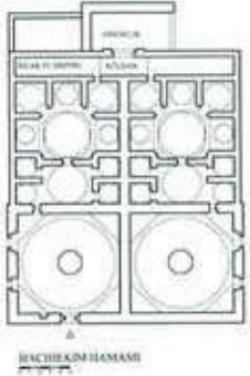
Şek. 19. Hacı Hakim Hamamı planı.
