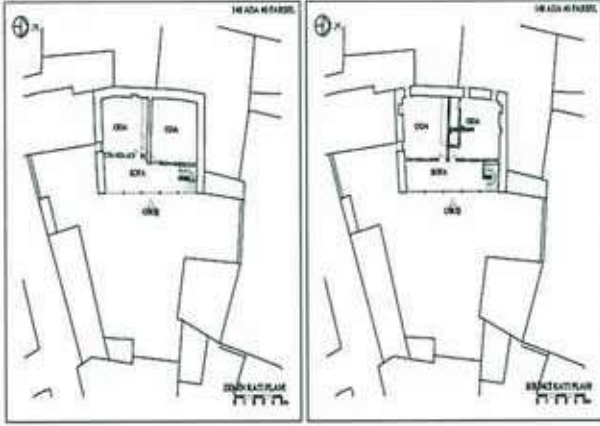
   . 5. D    sofabalı bir evin kat planları (env. no: J18.B5.1144)
