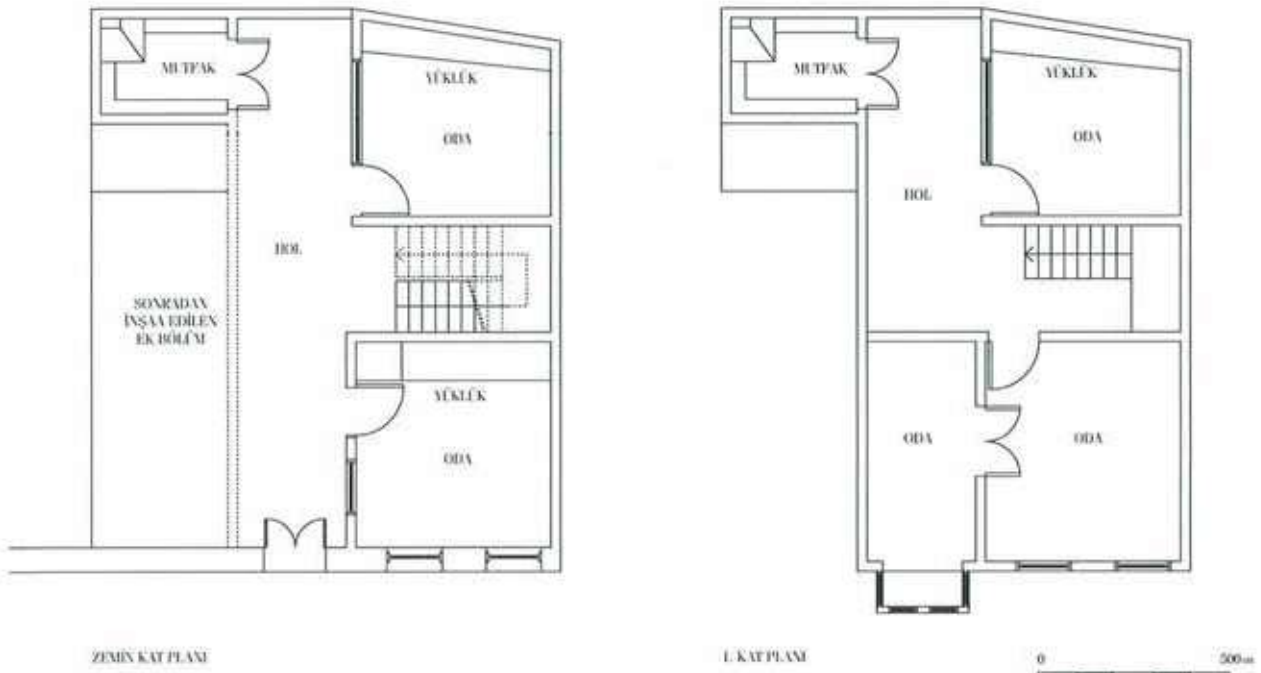
Şek. 16. 117 ada, 17 parselde (839. Sokak no. 23) bulunan konutun (env. no: L18B168) plan krokisi.
