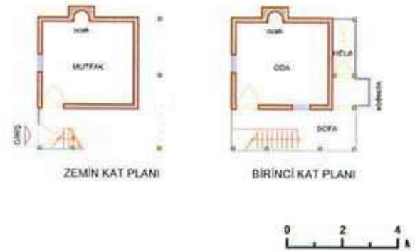
Şek. 12. Hüseyin Altan bağ evi kat planları.
