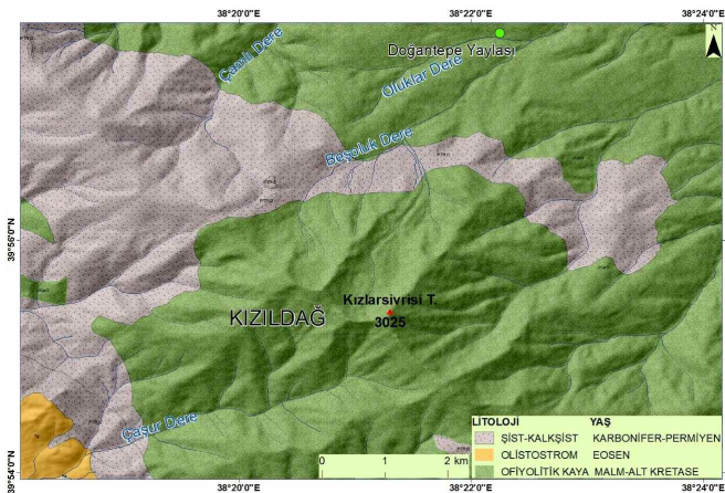
Şekil 3. Çalışma sahasının jeolojisi haritası (MTA'nın 1:25000 ölçekli jeoloji haritasından oluşturulmuştur.)
