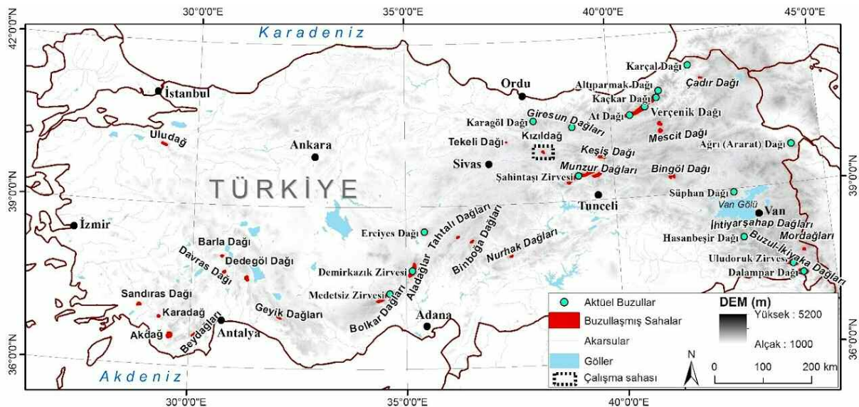
Şekil 1. Türkiye'de aktüel buzulların yer aldığı dağlar ve Kuvaterner'de buzullaşmaya uğramış alanlar (Bayrakdar vd., 2015'den değiştirilerek). Figure 1. The mountains harbouring active glaciers and glaciated mountains in Quaternary in Turkey (modified from Bayrakdar et al., 2015).
