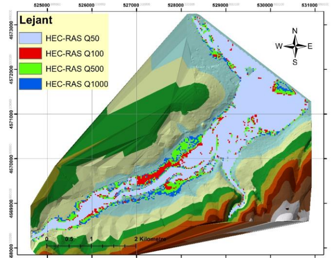
Şekil 2. HEC-RAS 2D taşkın yayılım haritası
