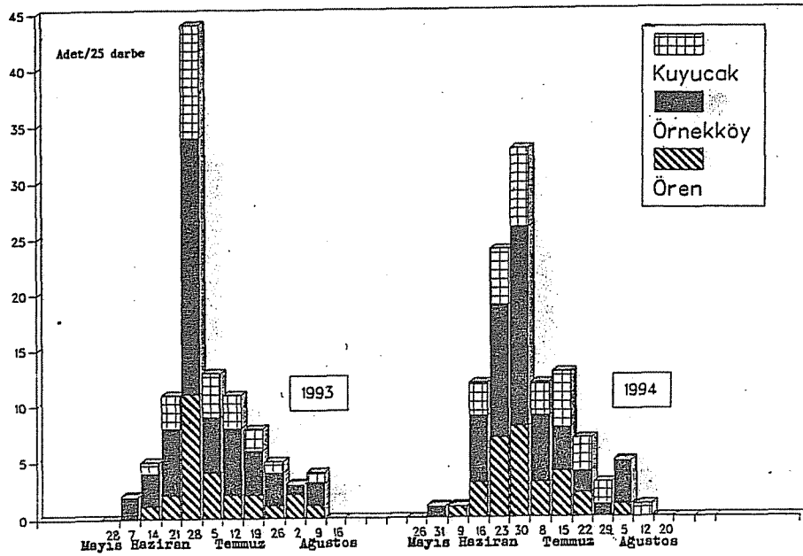
Şekil 4. Agrilus roscidus erginlerinin 1993 ve 1994 yıllarındaki sayısal değişimi
