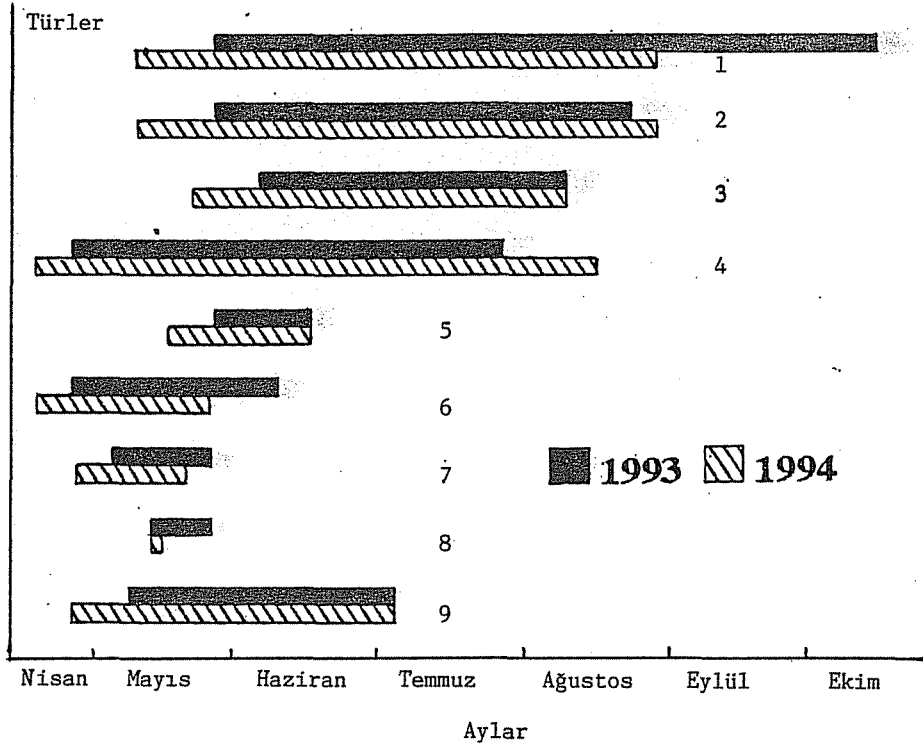
Şekil 6. Türlerin vegetasyon süresi içindeki dağılışları (1. C. tenebrionis , 2. C. carbonaria , 3. A. roscidus , 4. S. simulatrix , 5. A. nitidula signaticollis , 6. A. lugubris , 7. P. flavoguttata , 8. C. stigmatica 9. C. affinis ).
