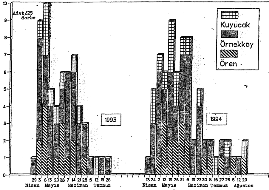
Şekil 5. Sphecoptera simulatrix erginlerinin 1993 ve 1994 yıllarındaki sayısal değişimi
