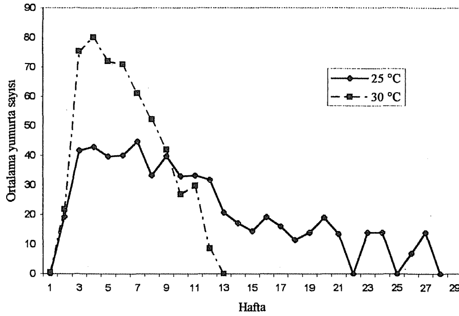
Şekil 1. Graphosoma semipunctatum 'un 25 ve 30°C'da bıraktıkları ortalama yumurta sayılarının haftalara göre dağılımı.
