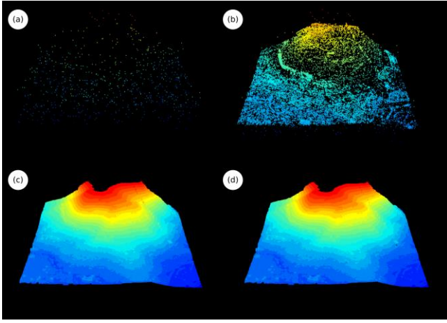
Şekil 2. Uyuşumsuz noktaların filtrelenmesi a) IVF filtreleme sonrası uyuşumsuz noktalar, b) SOR filtreleme sonrası uyuşumsuz noktalar, c) IVF sonrası temiz nokta bulutları, d) SOR filtreleme sonrası temiz nokta bulutları.
