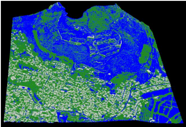
Şekil 3. Yer ve yer üzeri noktaların sınıflandırılması
