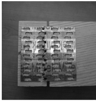
Şekil 5. Plaka kırılması
