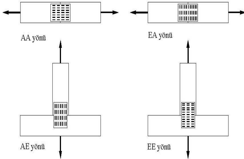
Şekil 3. Emniyet yüklerinin belirlenmesinde kullanılan dört yönlü test metodu.
