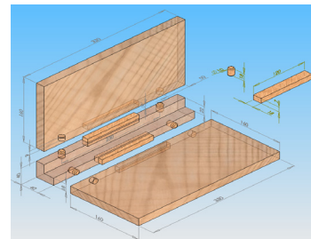
Şekil 1. L- köşe elemanlı karma birleştirme
