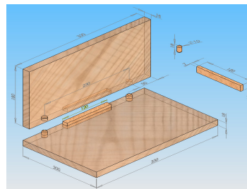
Şekil 2. Karma birleştirme
