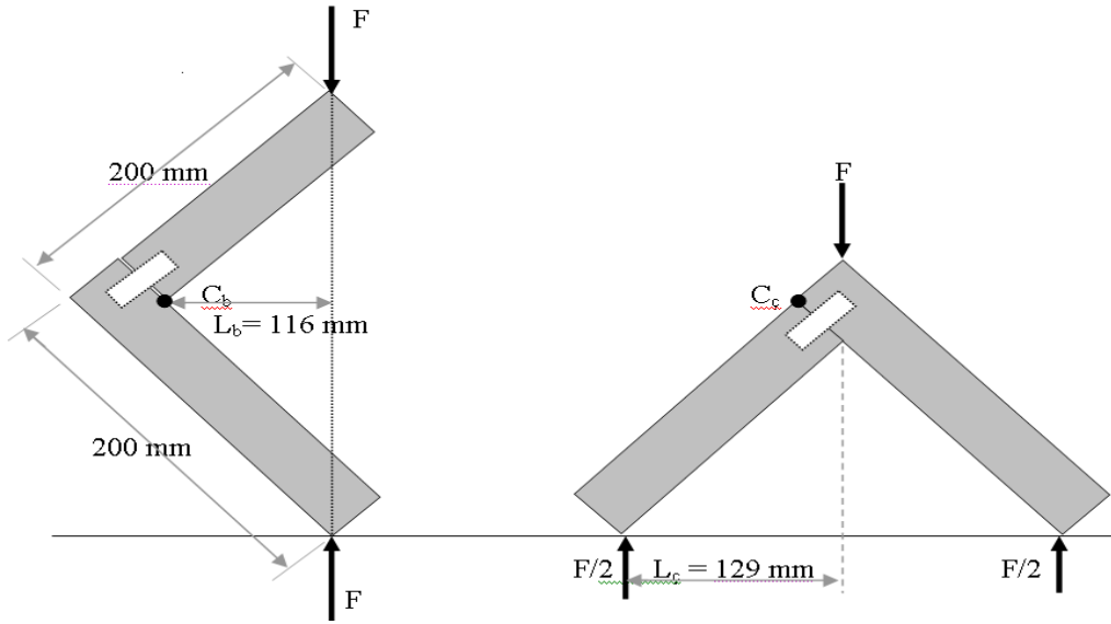
Şekil 3. Diyagonal basınç ve çekme testleri
