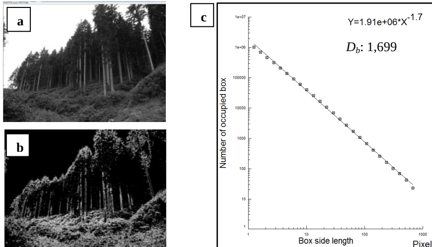
Şekil 4. Fotoğrafların fraktal boyutunun belirlenmesi süreci (a: orijinal fotoğrafın 8 bit olarak dönüştürülmesi, b: sınırların seçimi ve edit işleminin tamamlanması, c: Benoît fraktal analiz programı kullanılarak fotoğrafın fraktal boyutunun ( D_b ) hesaplanması).
