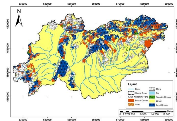
Şekil 2. Araştırma alanı arazi kullanım türü haritası
