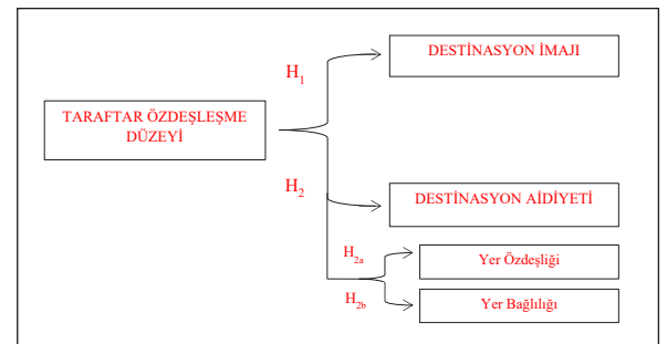
Şekil 1. Araştırmanın Modeli
