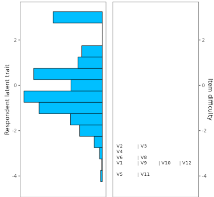
Şekil 2. Wright Haritası
