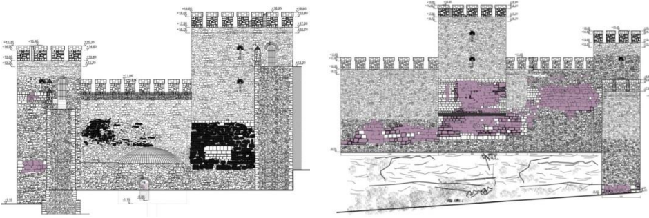
8 nolu dış kule ile 9 nolu dış kuleyi birbirine bağlayan batı duvarının içten görünüşü
