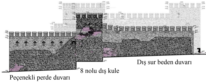
Çizim 3: 8 nolu dış kule özgün kabuk taşları ile bu kuleye saplanan duvarların görünüşü
