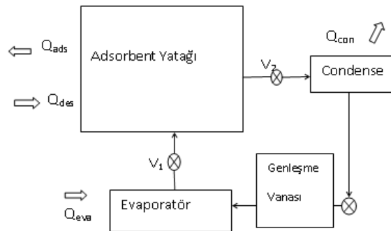
Şekil 2. Adsorbant yatağındaki enerji hareketleri
