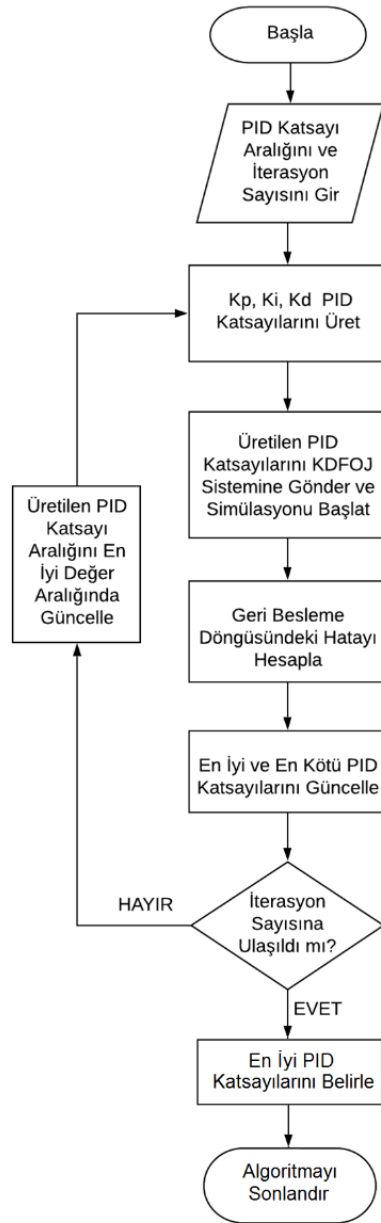
Şekil 3. Yerçekimi Arama Algoritması Akış Şeması
