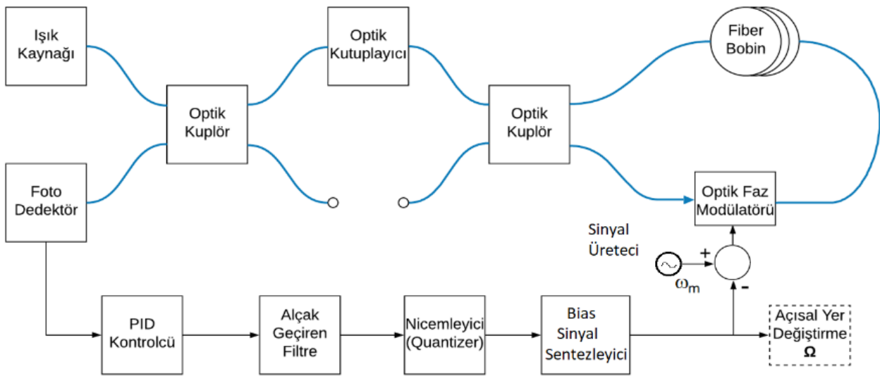
Şekil 1. KDFOJ Sisteminin Blok Diyagramı
