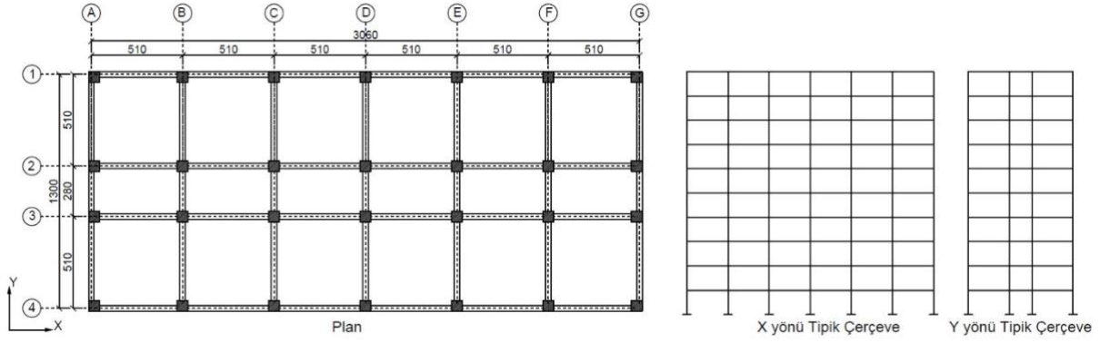
Şekil 1. Betonarme Çerçevesel Yapının Görünüşleri (Tüm ölçüler santimetre cinsindendir.)
