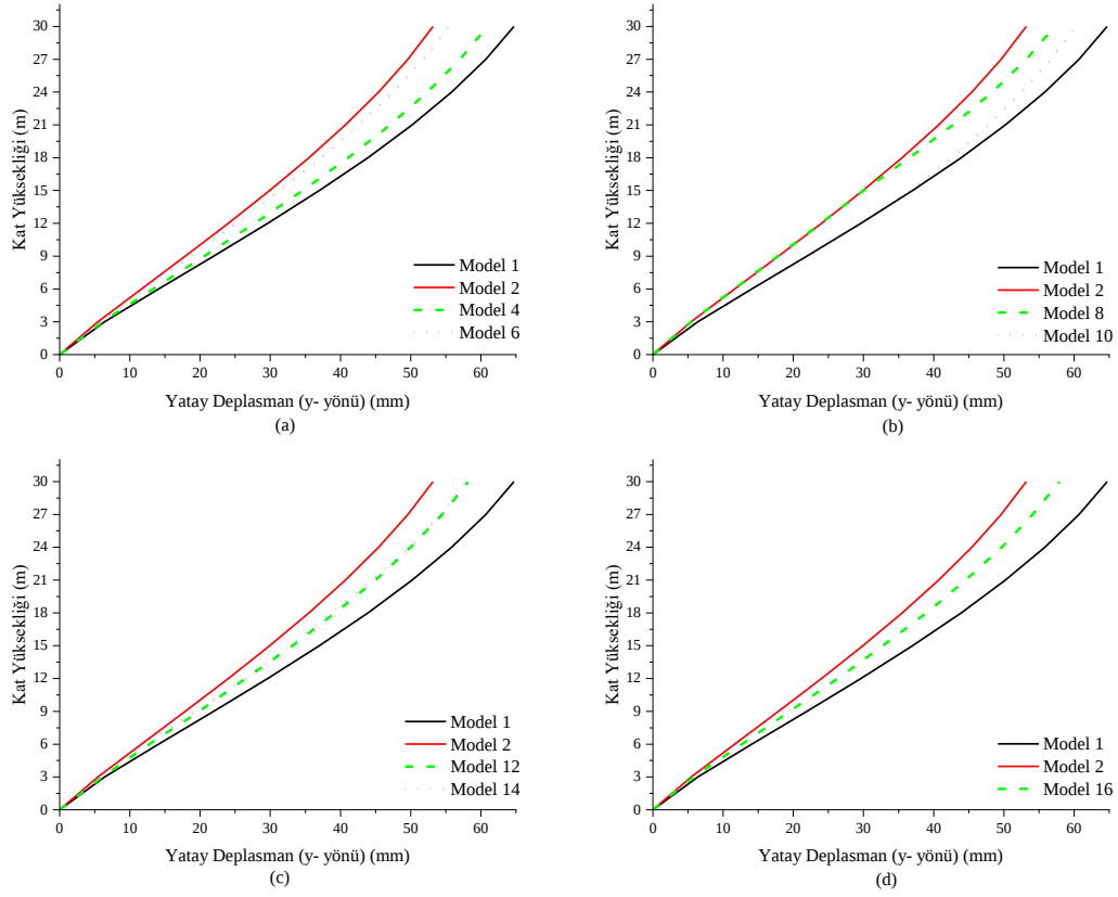
Şekil 7. Gazbeton Blok Kullanılan Modeller (y- yönü)
