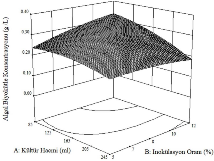
Şekil 2. C. vulgaris mikroalgal biyokütle üretimine ait kültür hacmi-inokülasyon oranı ikili etkileşimi için 3D grafiği
