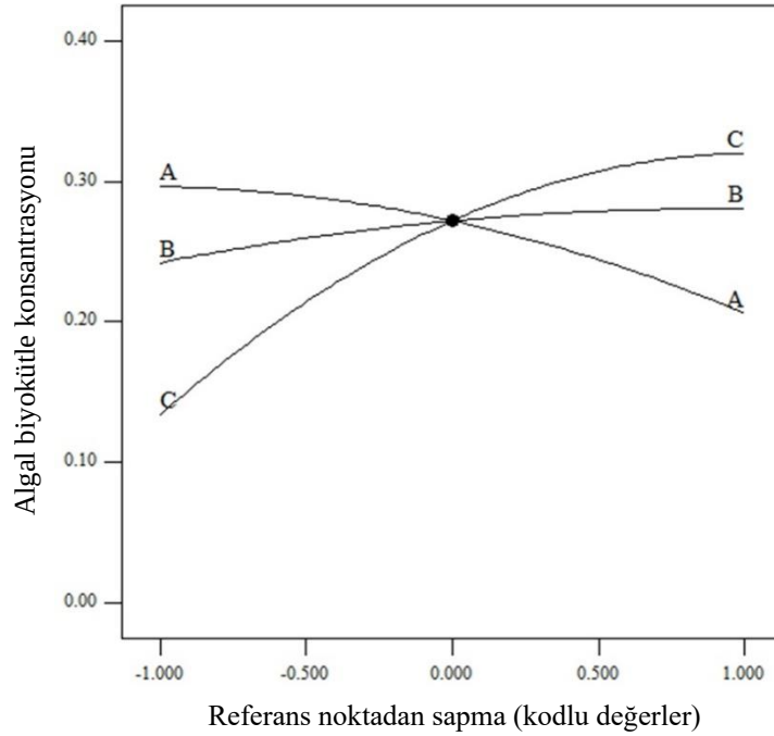
Şekil 3. C. vulgaris üretimi üzerine optimize edilen parametrelerin pertürbasyon grafiği
