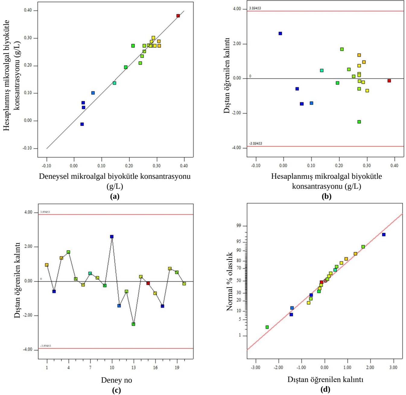
Şekil 1. RSM ile elde edilen bazı istatistiksel grafikler: (a) deneysel ve hesaplanmış mikroalgal biyokütle konsantrasyonlarının karşılaştırılması, (b) hesaplanmış mikroalgal biyokütle konsantrasyonu ile dıştan öğrenilen kalıntı değişimi, (c) deney no ile dıştan öğrenilen kalıntı değişimi, (d) dıştan öğrenilen kalıntı ile normal % olasılık değişimi.
