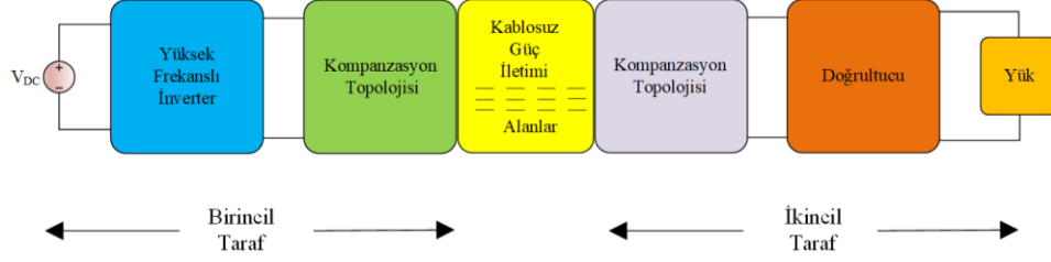
Şekil 1. Kablosuz güç transferinin genel bir yapısı.
