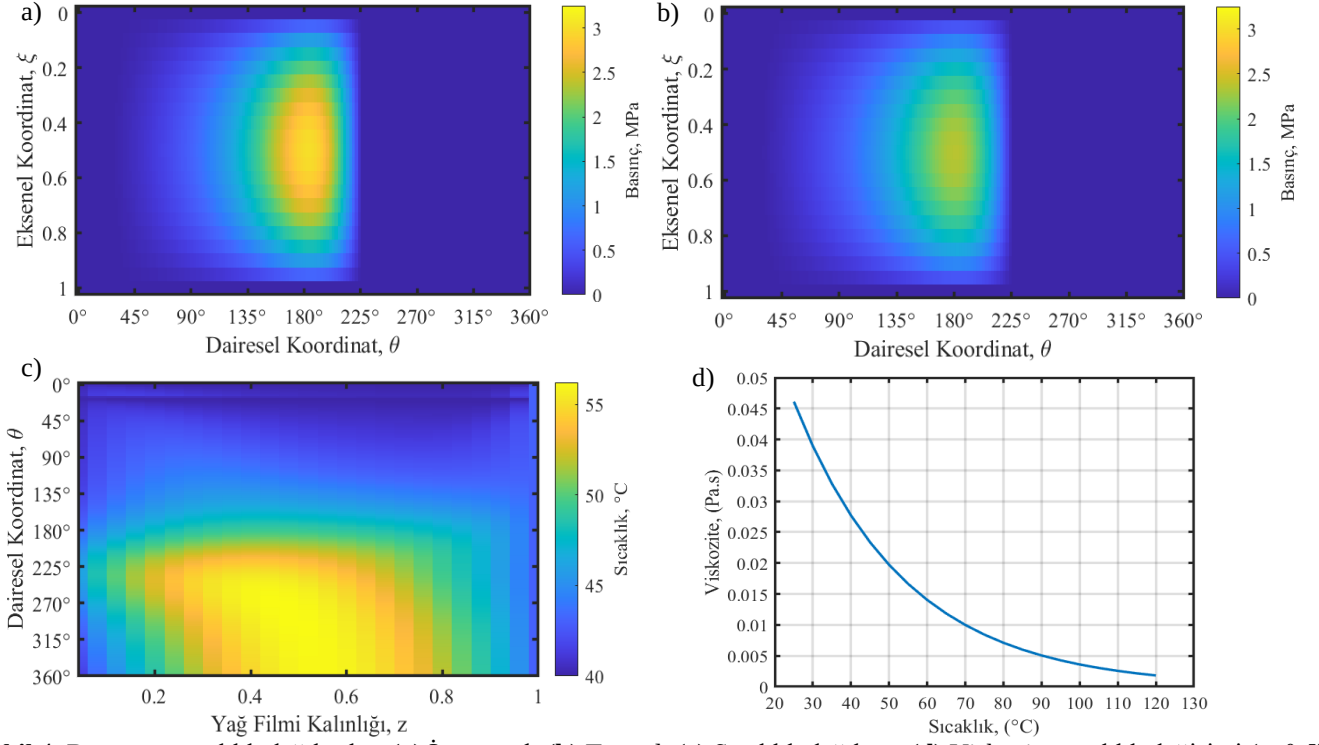
Şekil 4. Basınç ve sıcaklık dağılımları (a) İzotermal; (b) Termal; (c) Sıcaklık dağılımı; (d) Viskozite-sıcaklık değişimi ( \varepsilon=0.5 )
