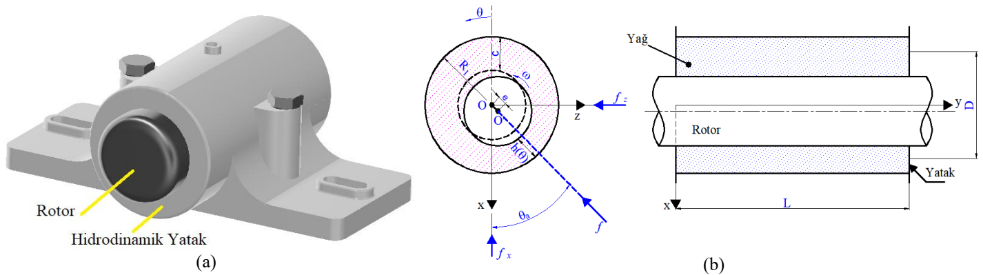
Şekil 1. Hidrodinamik yatak ile desteklenmiş bir rotor-yatak sistemi, a) izometrik görüntü, b) koordinat sistemi ve şematik görünüm
