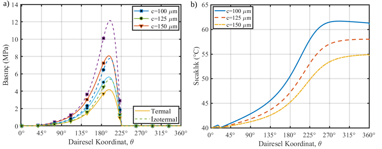
Şekil 5. Farklı radyal boşluk değerleri için yağ filminin (a) Basınç dağılımı; (b) Sıcaklık dağılımı ( \varepsilon=0.5 )
