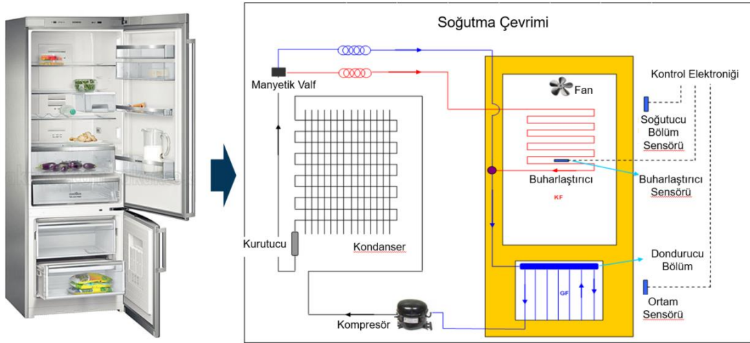
Şekil 1. Buzdolabı ve soğutma çevrimi
