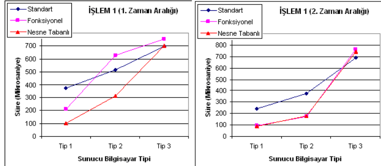
Grafik: 1 Veritabanına Kayıt Ekleme Örneğinden Elde Edilen Ortalamaların Faktörlere Göre Değişimi
