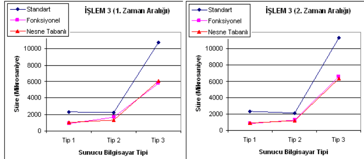
Grafik: 3 PNG Formathı Grafikler Üretme Örneğinden Elde Edilen Ortalamaların Faktörlere Göre Değişimi
