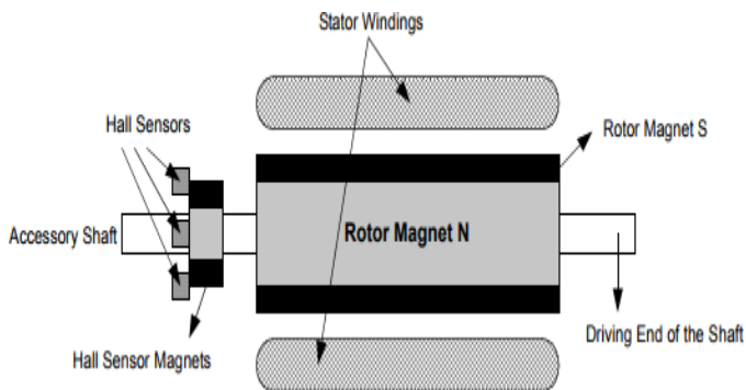
Şekil 1: Hallsensör bağlantısı
