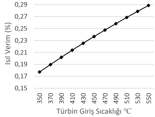
Şekil 3. Türbin giriş sıcaklığının değişiminin ısı verim üzerindeki etkisi
