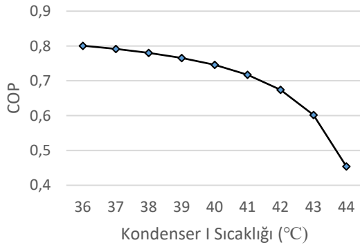
Şekil 10. Kondenser sıcaklığının atmasının COP üzerindeki etkisi
