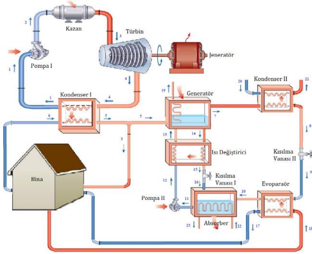
Şekil 1. Trijenerasyon sistemi
