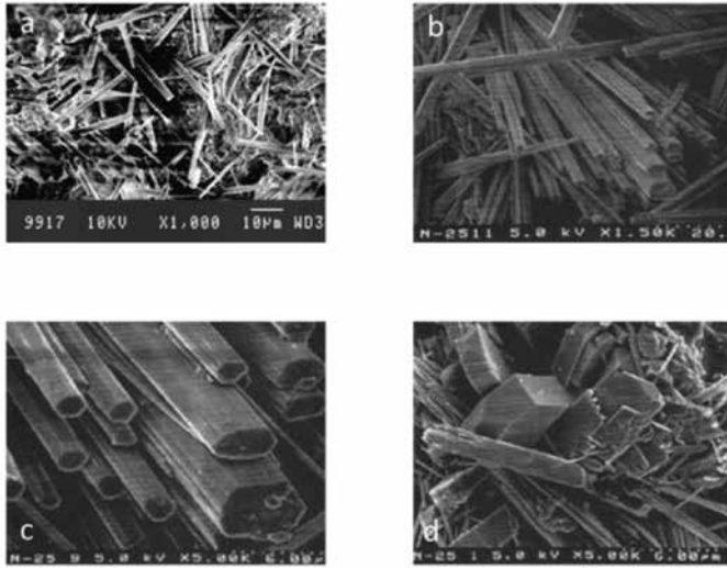
Şekil 8. A-Eriyonit Mineral İğneciklerinin Taramalı Elektron Mikroskop (SEM) Görüntüsü [22], B-Eriyonit Demetleri, C-Daha Fazla Büyütmeli Eriyonit Demetleri, D-Eriyonit (İğnems), Klinoptilolit, Kristobalit Mineralleri Birlikteliği [17], [20].
