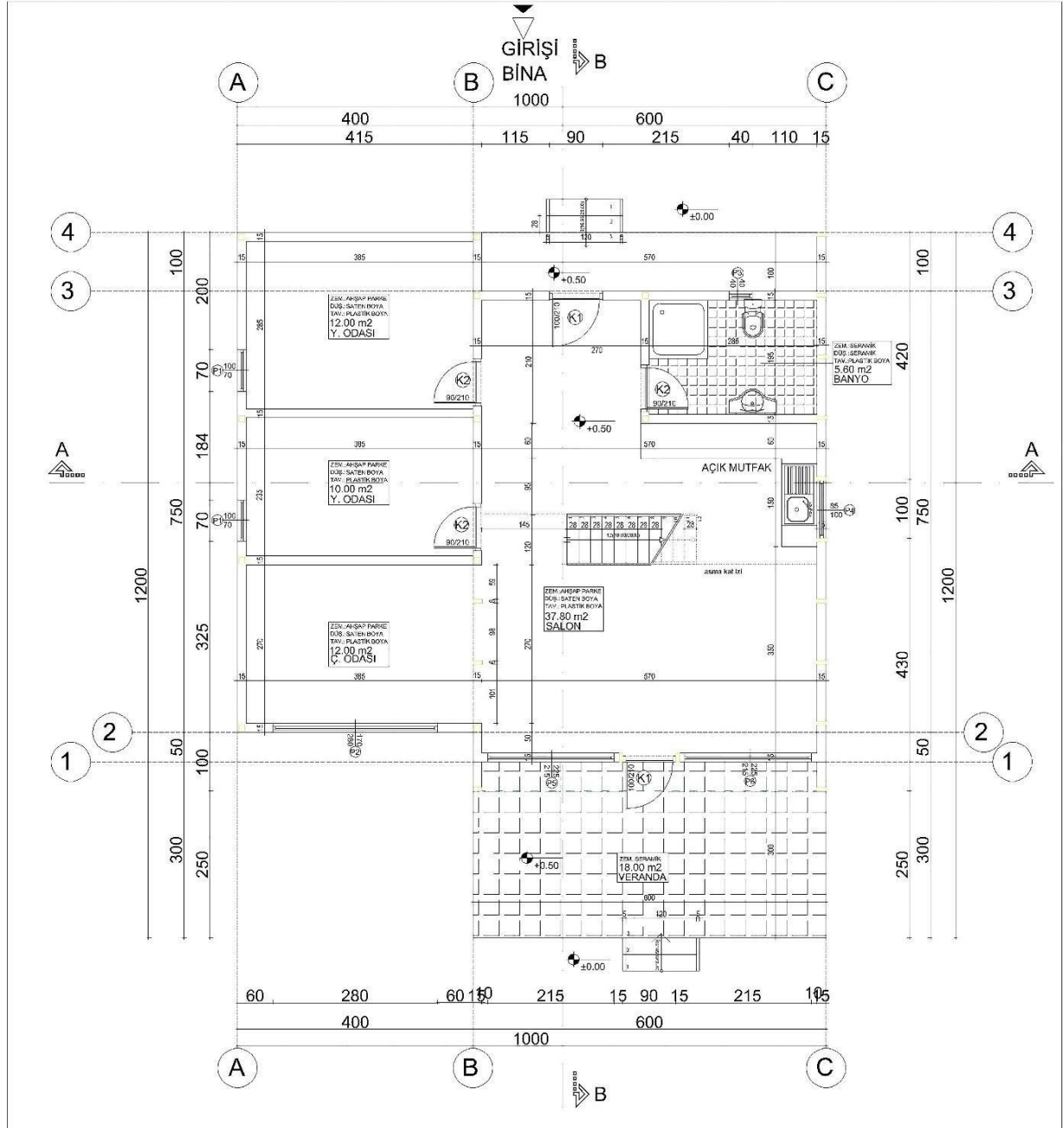
Şekil 2. Zemin kat planı (yazar arşivinden).
