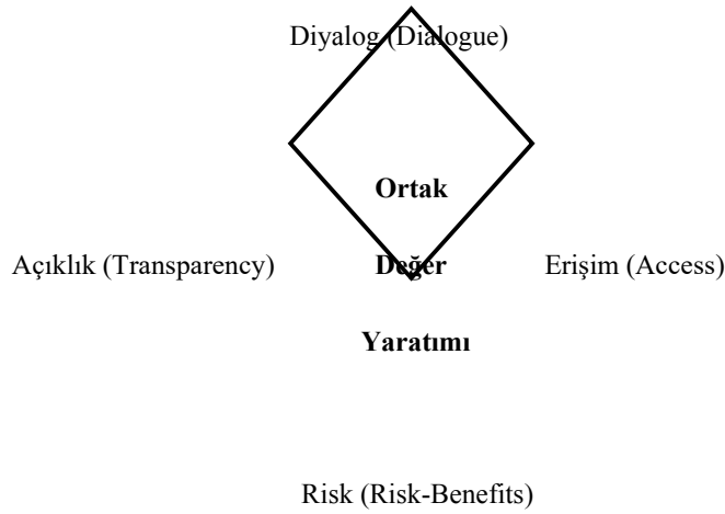
Şekil 2: Dart Modeli
