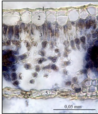
Şekil 6. Standart olarak kullanılan Huş ağacı yaprağı ( Betulae folium ) yaprak ayası enine kesiti: 1. Kütikula 2. Üst epiderma 3. Palizat parankiması 4. Sünger parankiması 5. Alt epiderma 6. Stoma.
