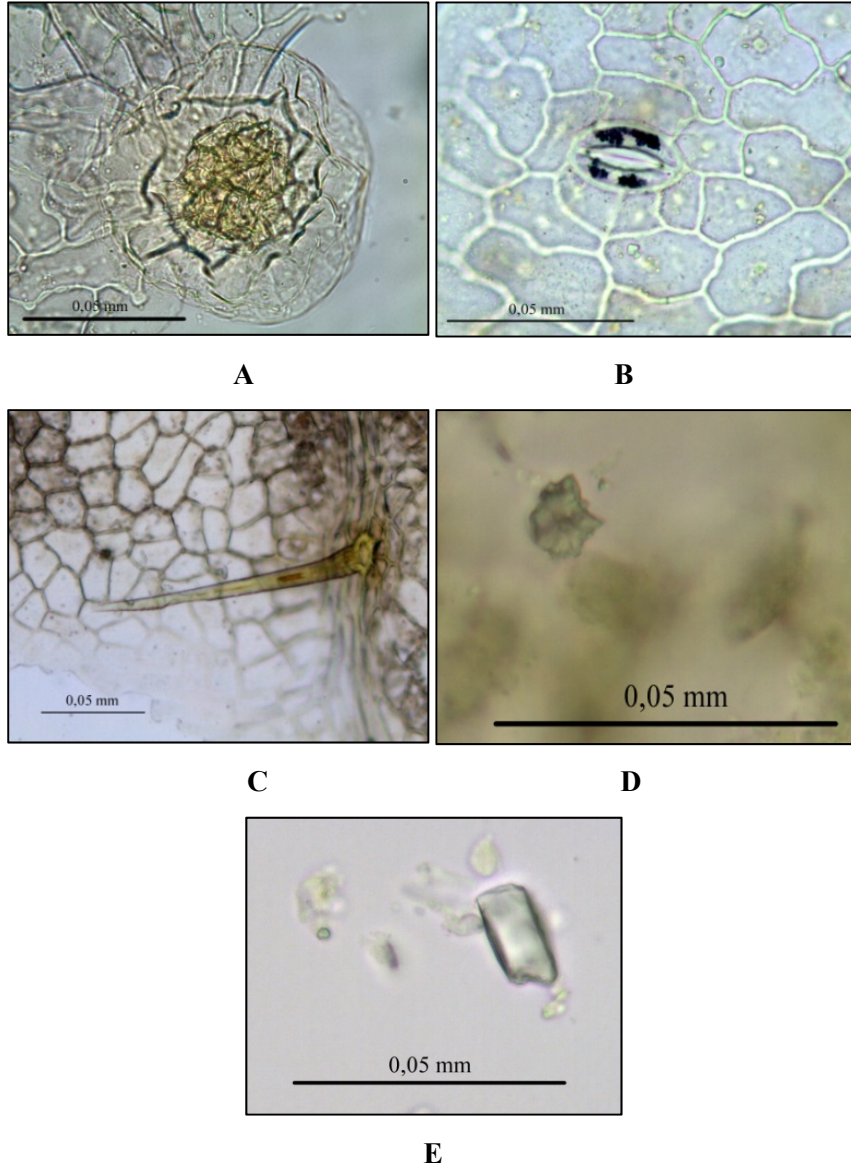
Şekil 9. Standart olarak kullanılan ve H1 kodu ile aktarlardan satın alınan huş ağacı yaprağı ( Betulae folium ) toz droğunun karakteristik elemanları: A. Peltat salgı tüyü B. Stoma C. Örtü tüyü D. Druz E. Basit billur.
