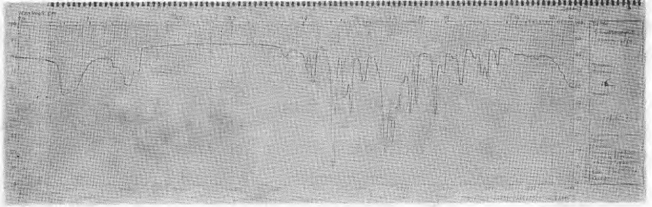
Spektr. 3. O. heterocarpus uçucu yağının IR spektrumu.
