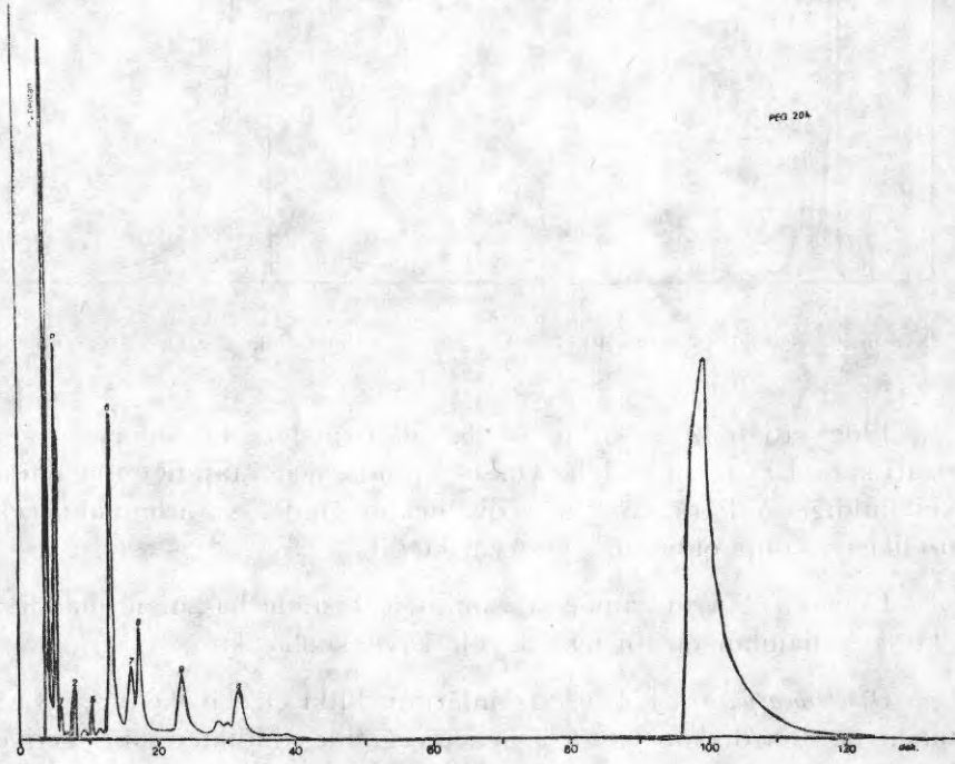
Krom. 9. G. urbanum uçucu yağının PEG 20M (160°C) kolonundaki gaz kromatogramı.
