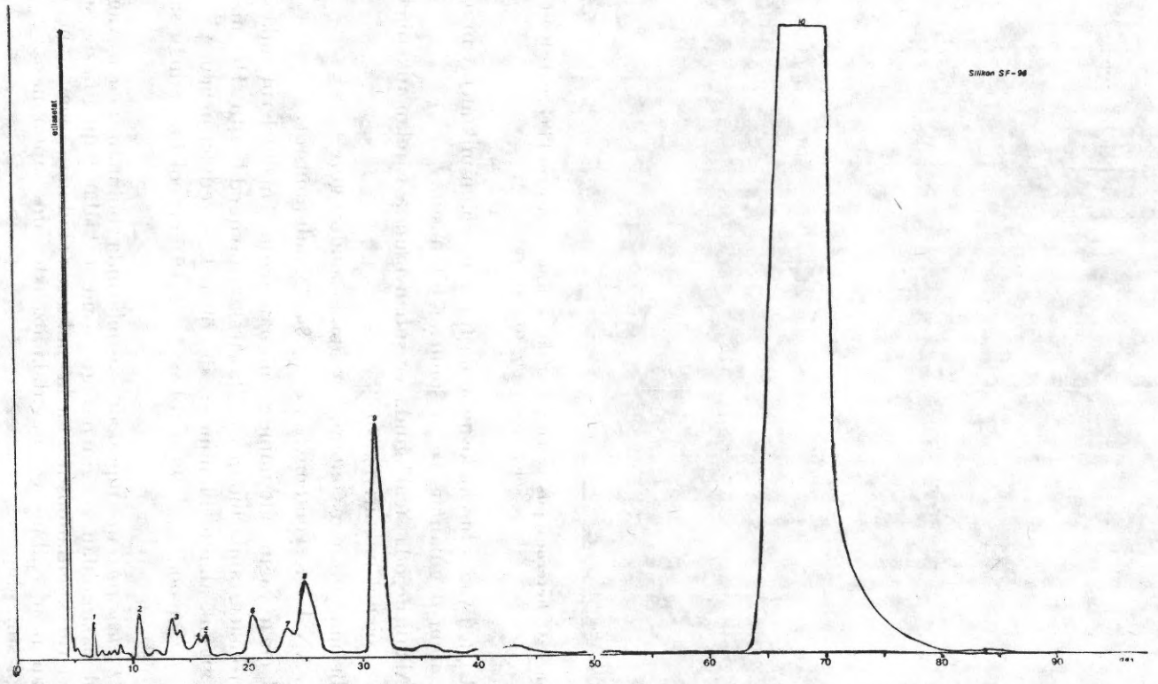
Krom. 8. O. heterocarpus uçucu yağındaki oksijenli bileşiklerin Silicon SF-96 kolonundaki gaz kromatogramı.
