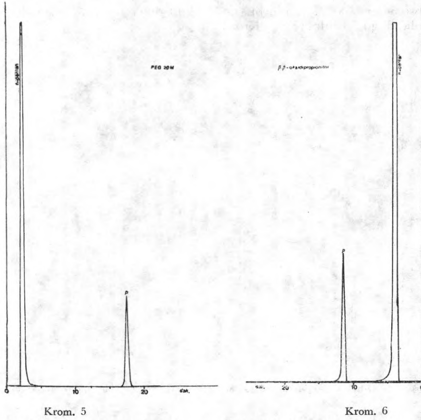
O. heterocarpus uçucu yağındaki monoterpenik hidrokarbürlerin 60°C de PEG 20M (Krom.5) ve 50°C de \beta,\beta' -oksipropionitril (Krom. 6) kolonlarındaki gaz kromatogramları.
