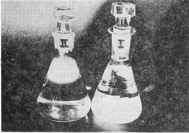
Resim 2. Polistiren yapısındaki A 825 E plastiği ile fosforlu pestitiser grubundan Dursban arasındaki etkileşme. I) A 825 E plastiği su içinde doğal granüler yapıyla. II) Aynı plastik Dursban. içinde iki ay zarfında jelleşerek kısmen pestisit içinde erimiş durumda, henüz erimemiş bölüm üst yüzeyde tabakalaşmış olarak.
