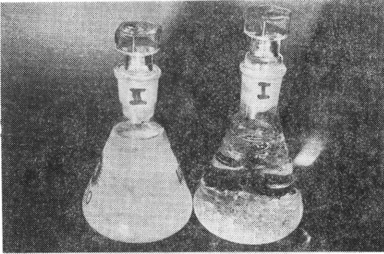
Resim 3. Polivinilklorür yapısındaki SE 9 plastiği ile klorlu pestitiser grubundan Korlin arasındaki etkileşme I) SE 9 plastiği su içinde doğal granüler yapıyla. II) Aynı plastik Korlin içinde iki ay zarfında şişerek hacmini kabın hacmine çıkarmış durumda.
