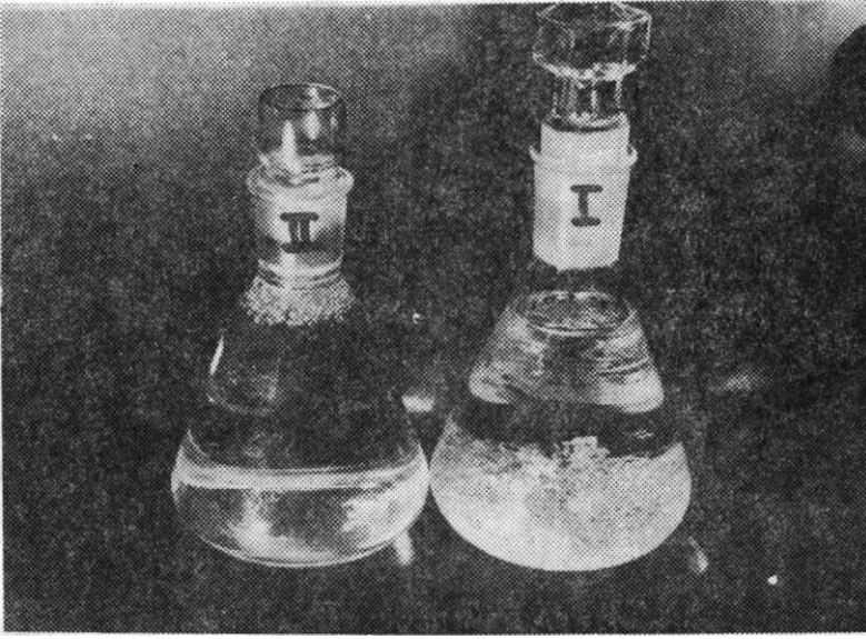
Resim 1. Polistiren yapısındaki K 500 plastik maddesi ile fosforlu pestisitler grubundan Rogor arasındaki etkileşim. I) K 500 plastiği 100 ml su içinde doğal granitler yapısı halinde dibe çökmüş olarak II) K 500 plastiği 100 ml Rogor içinde, iki ay zarfında jelleşerek kısmen pestisit içinde ermiş durumda, henüz erimemiş bölüm üst yüzeyde tabakalaşmış olarak.
