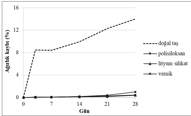
Şekil 6. Doğal ve iyileştirilmiş ŞT'nın asite karşı dayanım grafiği
