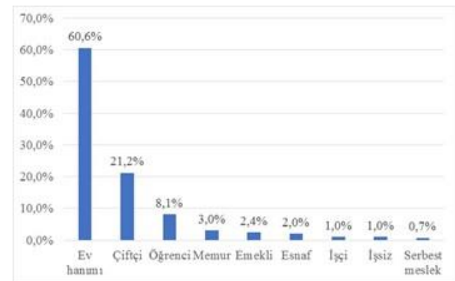
Şekil 3. Katılımcıların meslekleri
