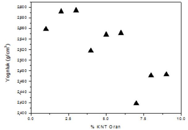
Şekil 1. Farklı sıcaklıklarda sinterlenen ve oranlarla takviyeli AlMg/KNT kompozit numunelerin yoğunluk değişimleri
